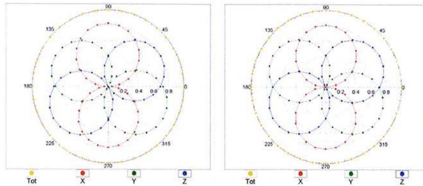
f=1800 MHz,R22
